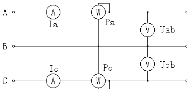
图二十、三相三线计量原理图
