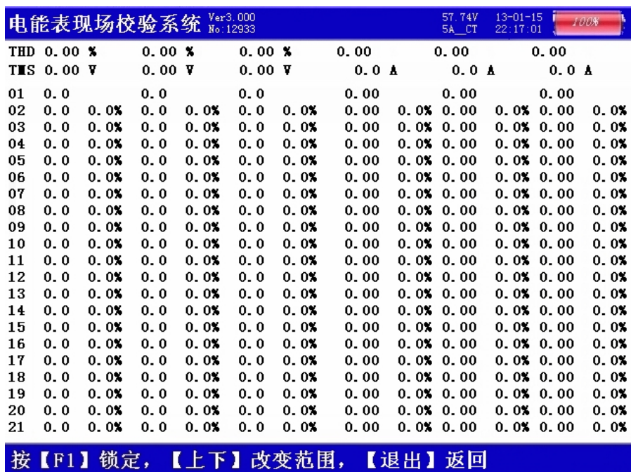
图十八、谐波测试屏
