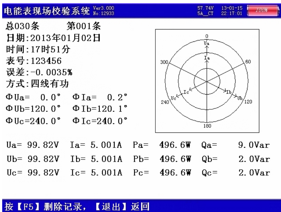
图十九、历史数据屏
